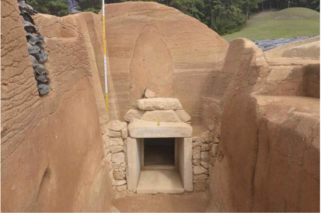
<그림 9. 부여 왕릉원 4호분 돌방과 봉분의 층위>
