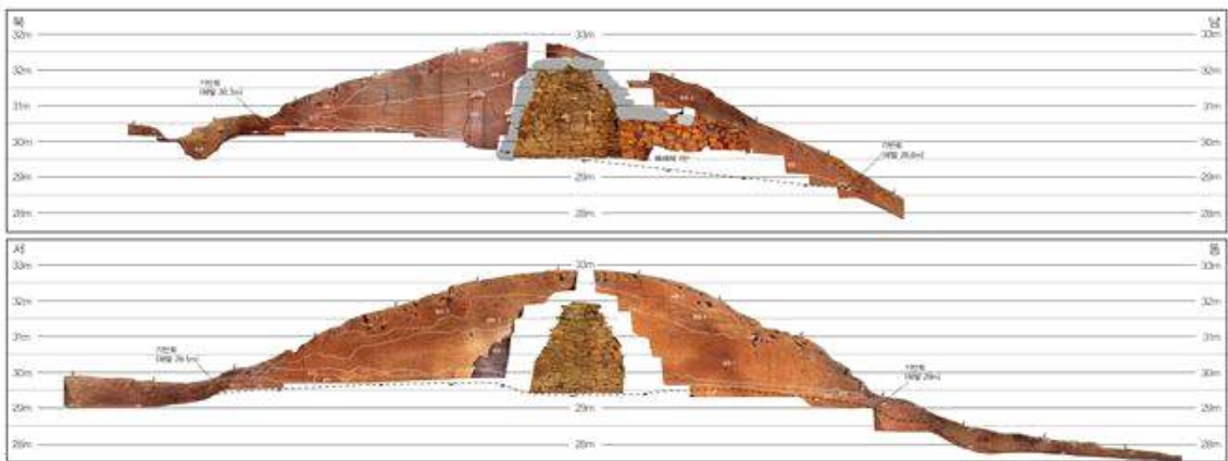
<1호분 단면도>
