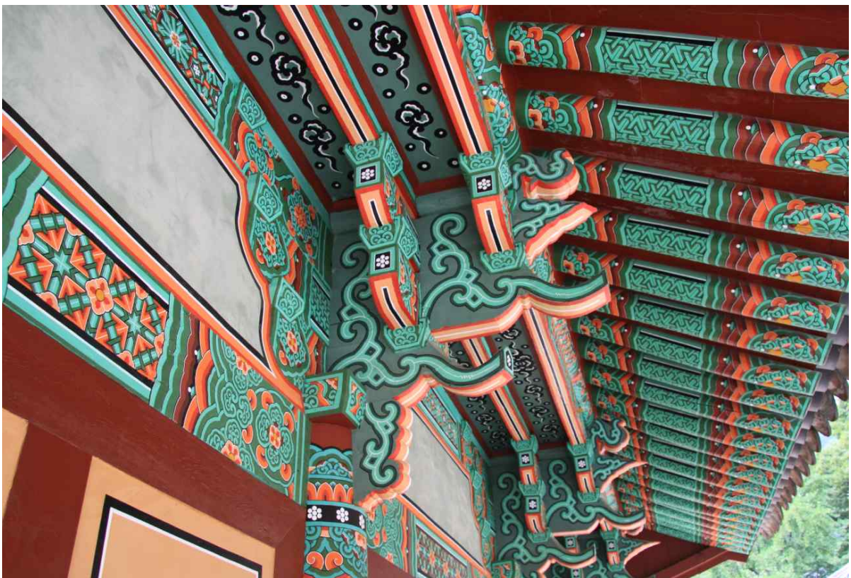
<공포 - 배면>
