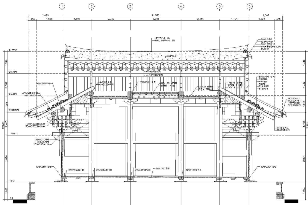
극락전 횡단면도
