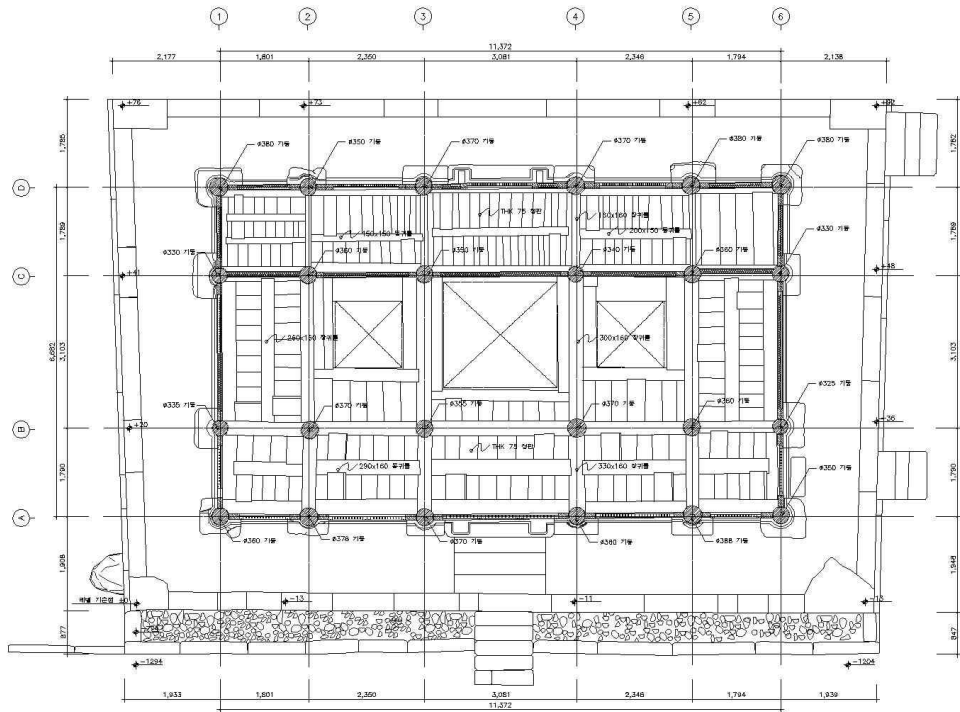
극락전 평면도
