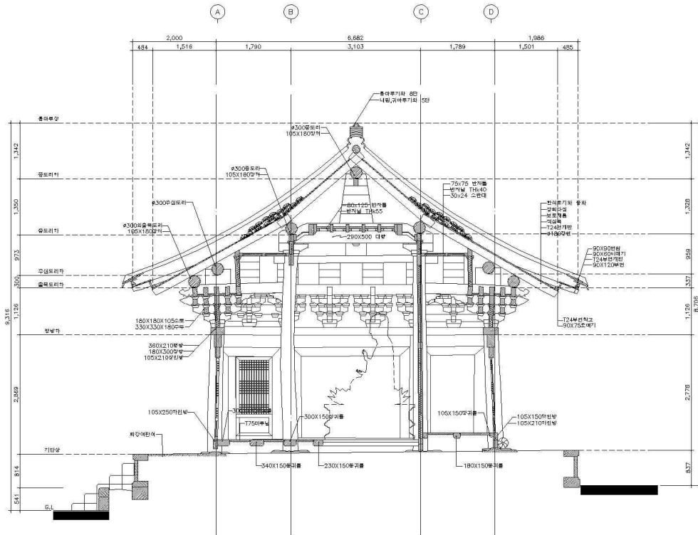
극락전 종단면도
