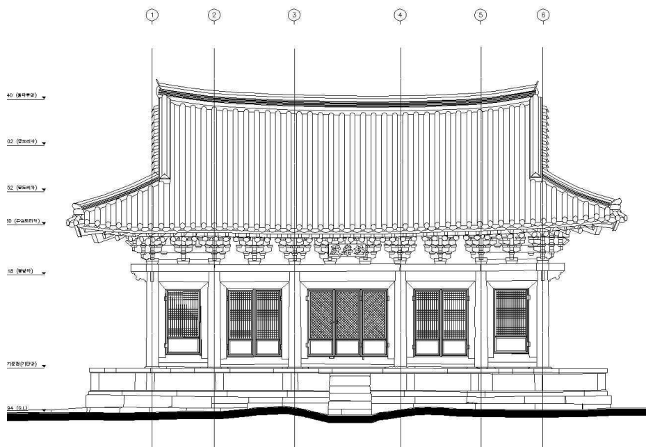
극락전 정면도
