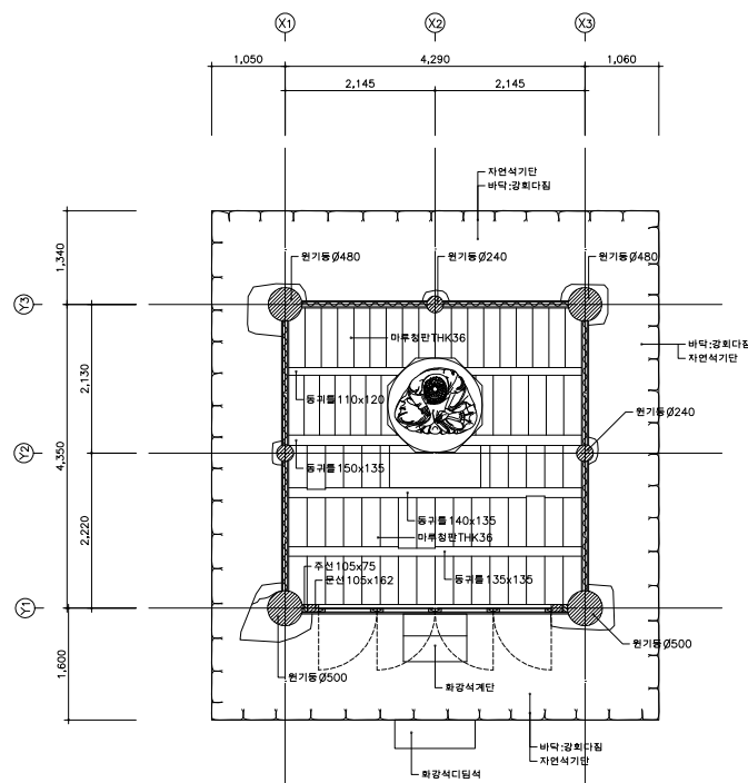
수마제전 평면도
