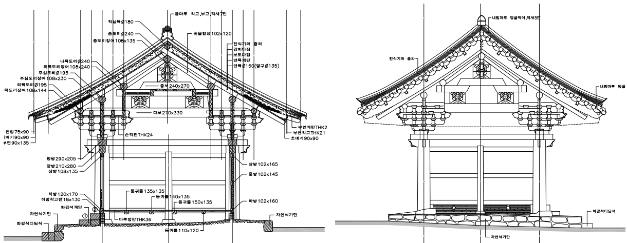
수마제전 중단면도
