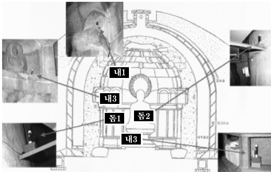
석굴암 석굴 및 이중돔내 온·습도 센서
