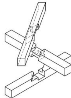
32-1. 6모3분턱
