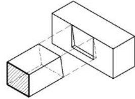
34. 빗턱맞춤
