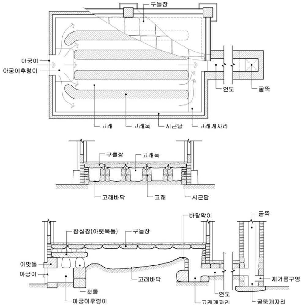
온돌의 구조(함실아궁이-궁궐)
