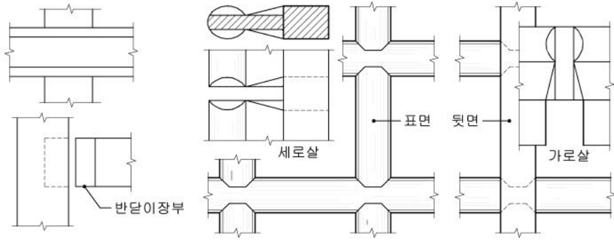
반달이장부맞춤
