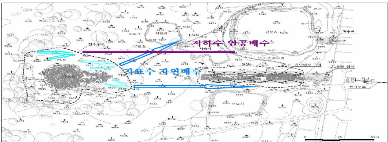
<홍낭시다 주신전 주변 지형/집수 현황도 및 배수개념도>
