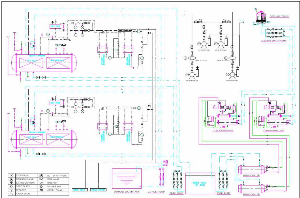
대형 진공동결건조기 계통도(10m, 나주시 천연색소산업화지원센터 식품 건조용)
