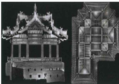
▲ 3D 스캔 및 모델링 데이터 제작 (17년 수원화성)
