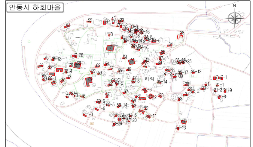
도면1. LPG배관망 신청세대
