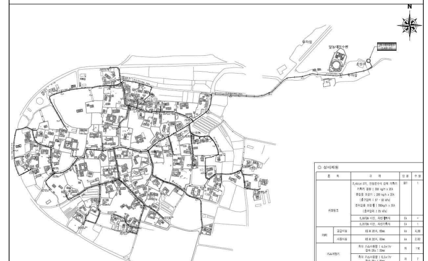
도면2. LPG배관망 구축 계획도
