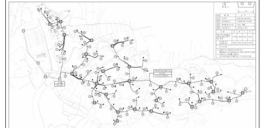
통신망 공사 계획도
