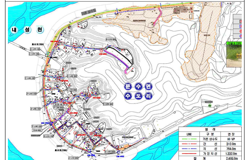
상수도관 교체 계획도
