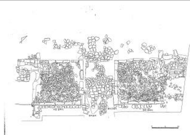
진해루지 발굴조사 도면
